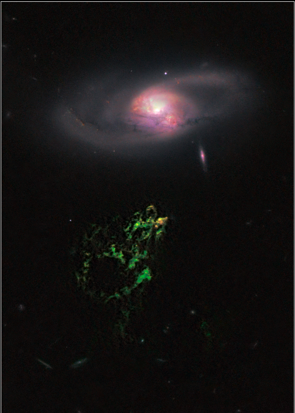
Hanny's Voorwerp Hubble Space Telescope WFC3 ACS ■ WIYN
