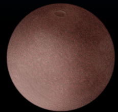
2005 FY9
