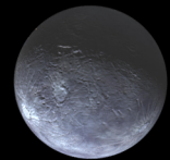
Quaoar
