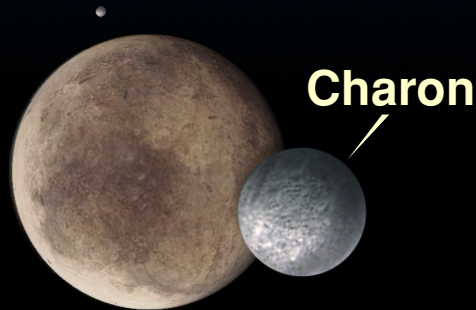
Pluto
