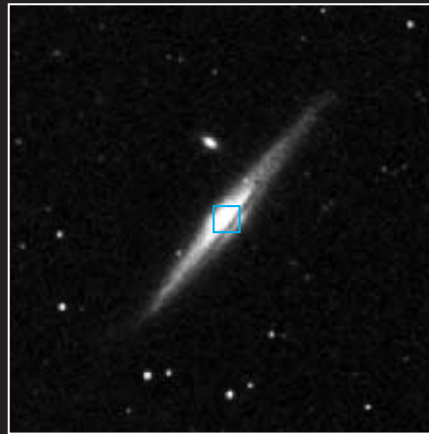
NGC 5965
