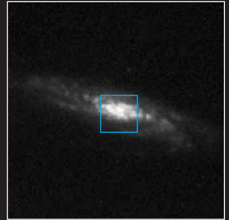
NGC 7537
