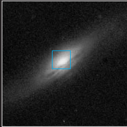
NGC 5689
