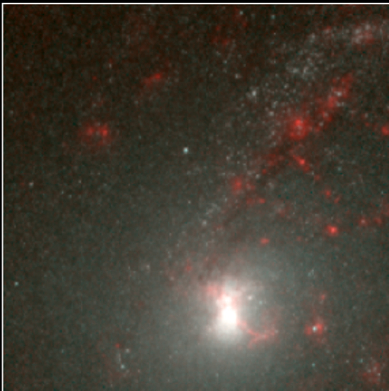
NGC 6946
