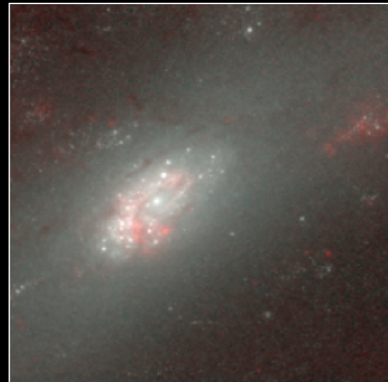
NGC 2903
