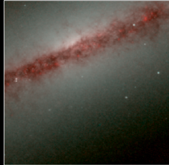
NGC 891
