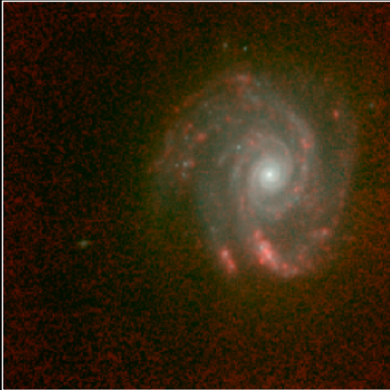
NGC 5653
