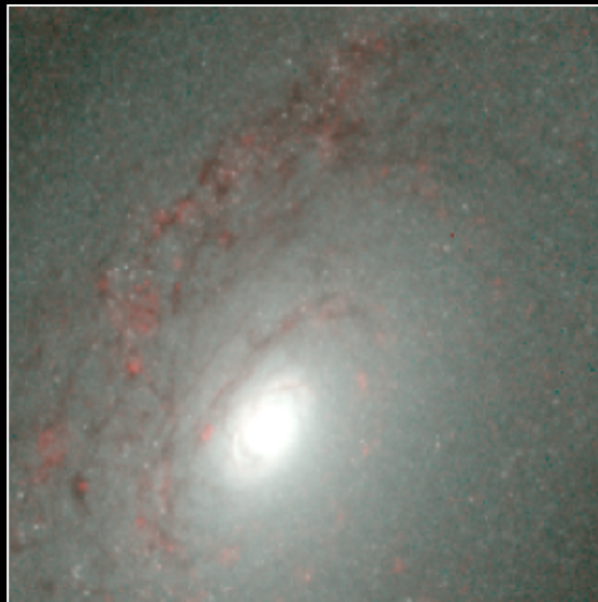
NGC 4826
