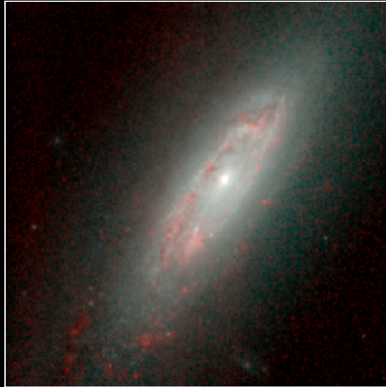
NGC 3593
