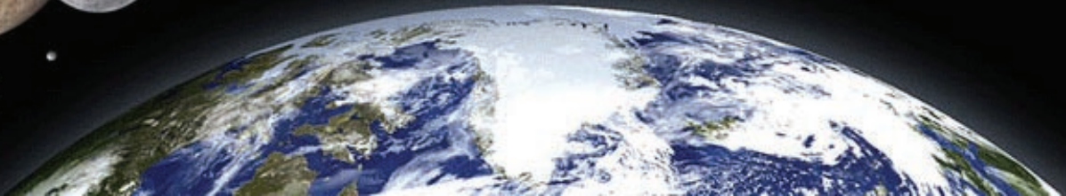
Earth
