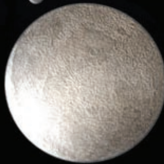
Eris
